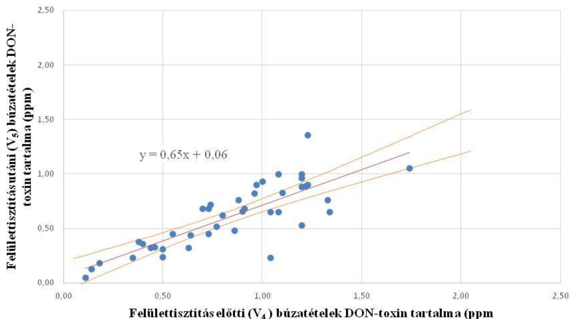
4.27. ábra Schule Verticone VPC 480 felülettisztító gép előtt (V 4 ) és után (V 5 ) megszedett minták regressziós függvénye 2013. évjárat adatai alapján
