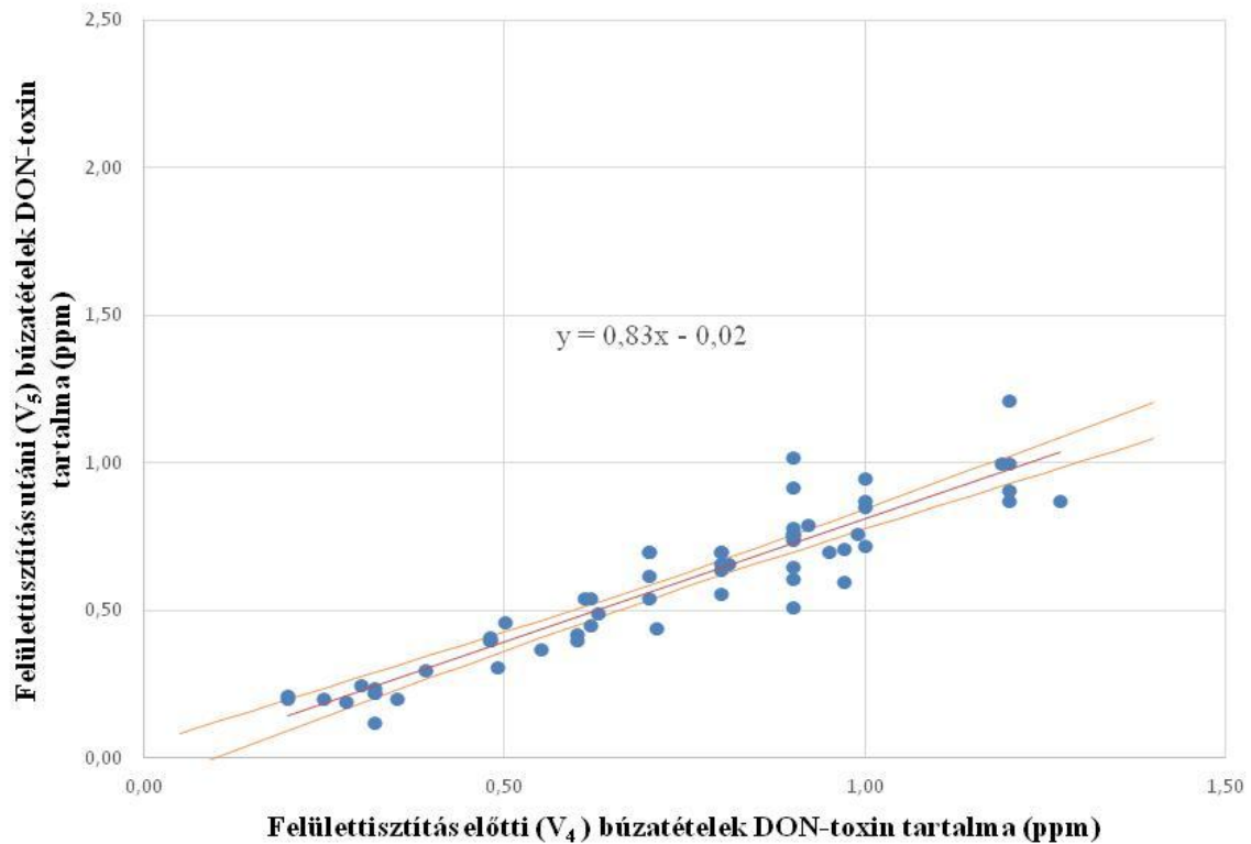
4.30. ábra Schule Verticone VPC 480 felületisztító gép előtt (V 4 ) és után (V 5 ) megszedett malmi búza minták regressziós függvénye 2015. évjárat adatai alapján
