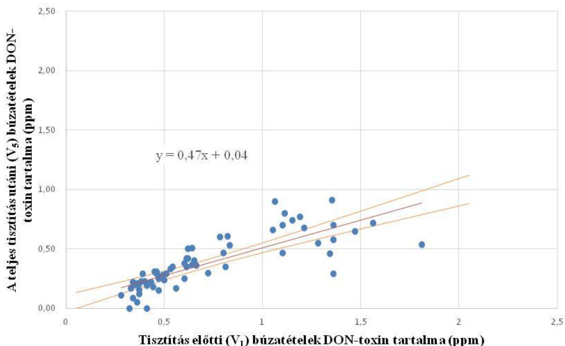
4.33. ábra A malmi búzátételek kiinduló DON-toxin koncentrációjának ( V_1 ) és a teljes tisztítási folyamatot követően ( V_5 ) mért toxintartalom regressziós függvénye a 2014. évjárat adatai alapján
