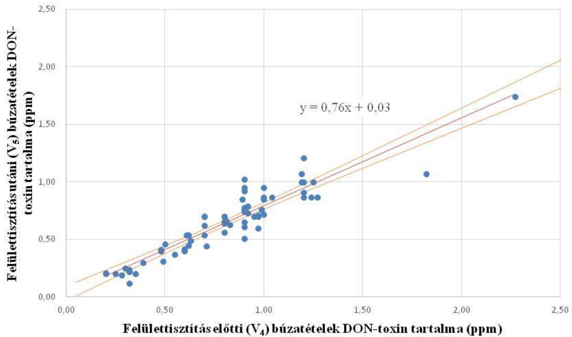
4.29. ábra Schule Verticone VPC 480 felületisztító gép előtt (V 4 ) és után (V 5 ) megszedett 70 mintából képzett regressziós függvény 2015. évjárat adatai alapján
