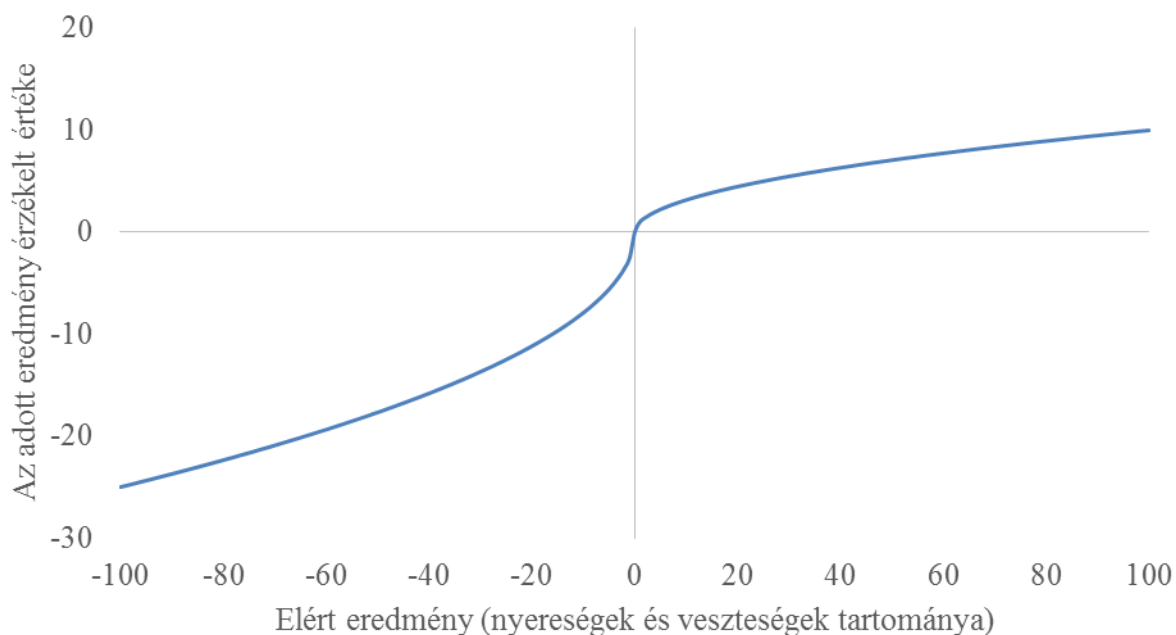
1. ábra: A kilátásmélet értékfüggvénye
